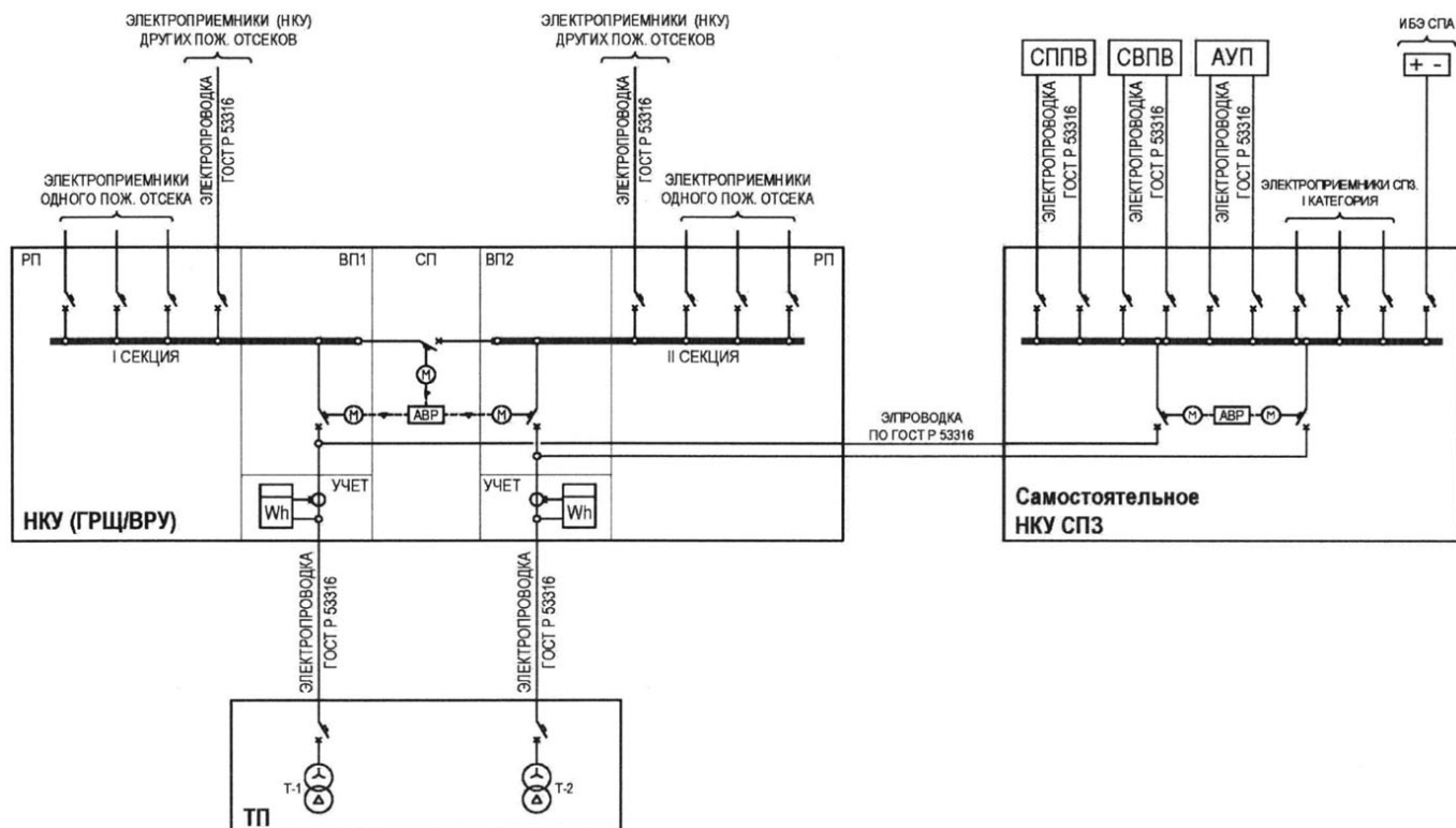
Рисунок А.2. Структурная схема организации электроснабжения электроприемников I категории надежности и применении самостоятельного НКУ СПЗ
