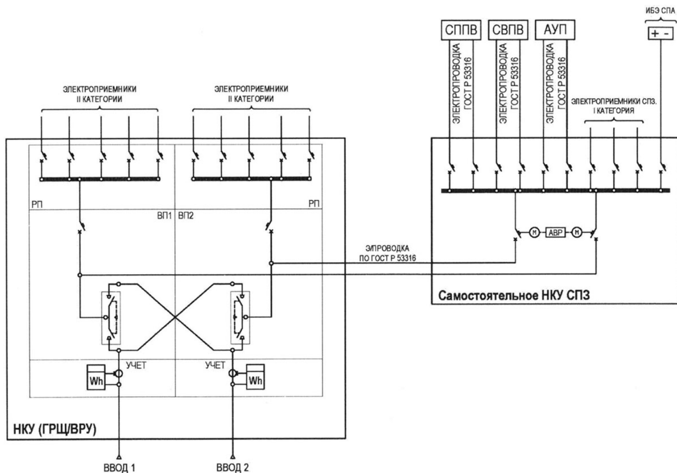
Рисунок А.4. Структурная схема организации электроснабжения электроприемников II категории надежности и применении самостоятельного НКУ СПЗ
