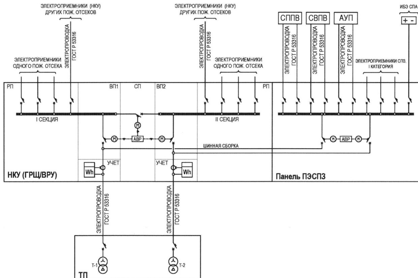
Рисунок А.3. Структурная схема организации электроснабжения электроприемников I категории надежности и применении панели ПЭСЗ3 в составе многопанельного НКУ
