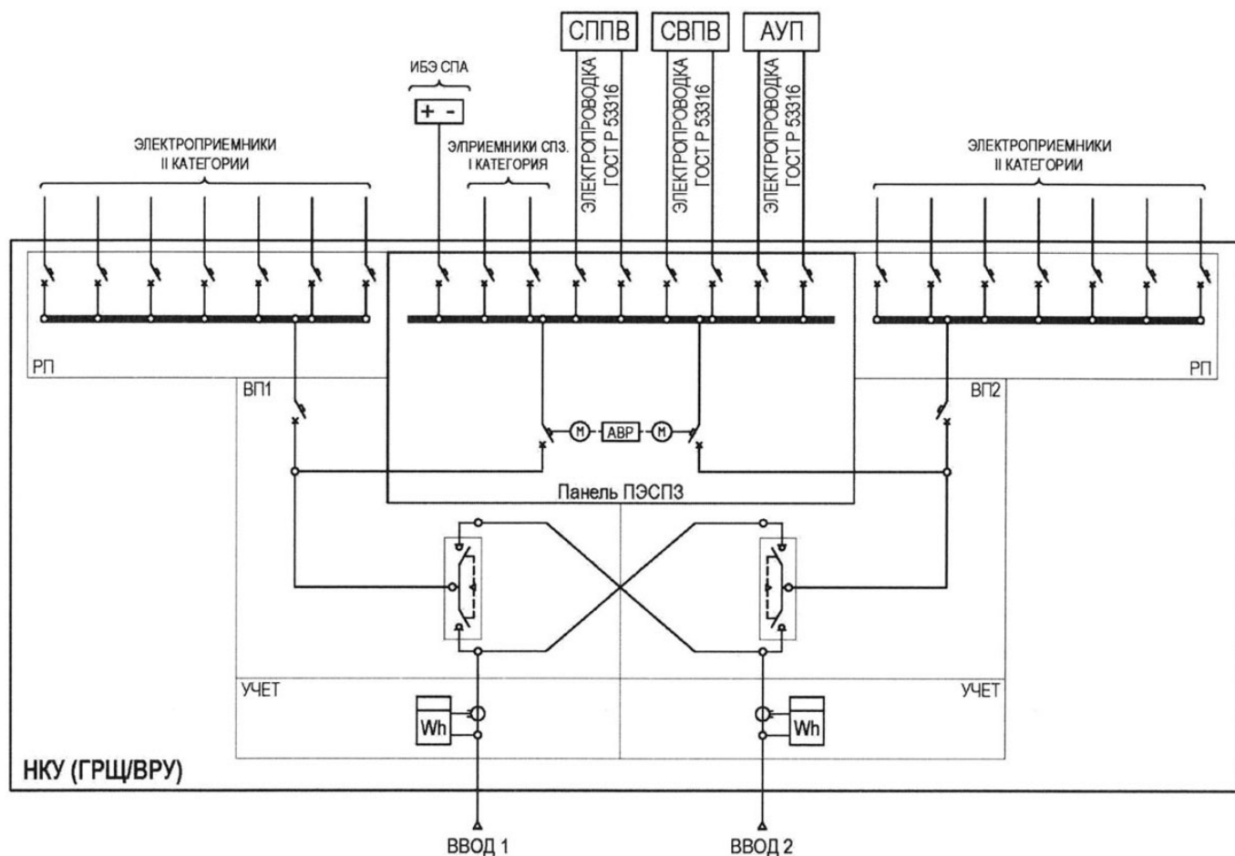
Рисунок А.5. Структурная схема организации электроснабжения электроприемников II категории надежности и применения панели ПЭСЗ в составе многопанельного НКУ
