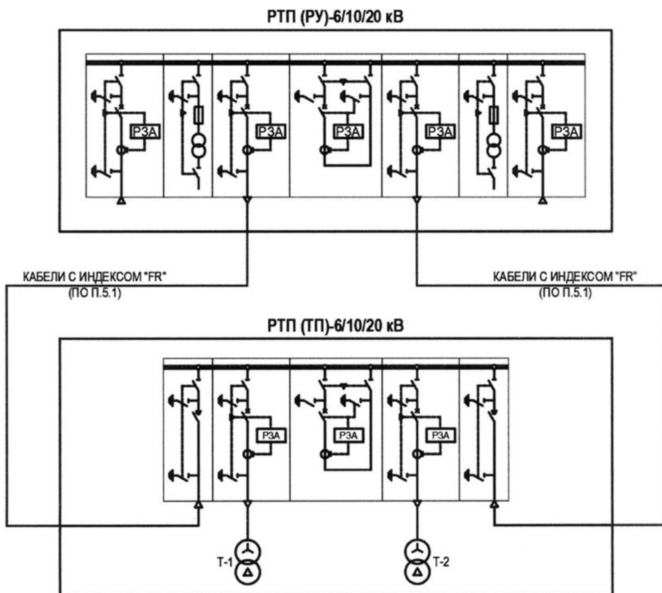
Рисунок А.1. Структурная схема организации электроснабжения при размещении ТП на
