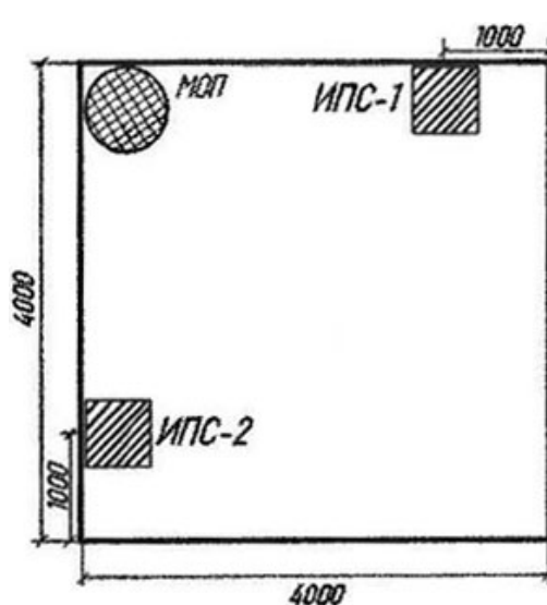
з) ИП сателлитный тепловой (ИПС-1-2)
