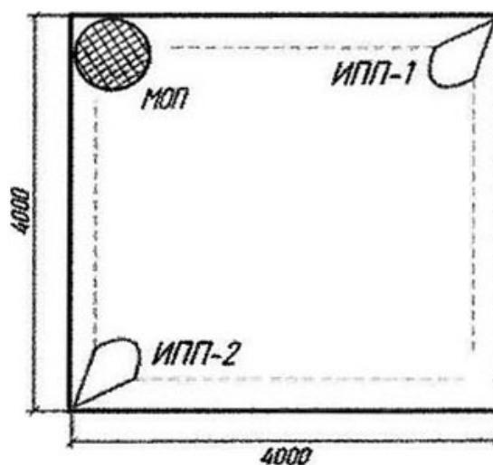
е) ИП пламени (ИПП-1-2)
