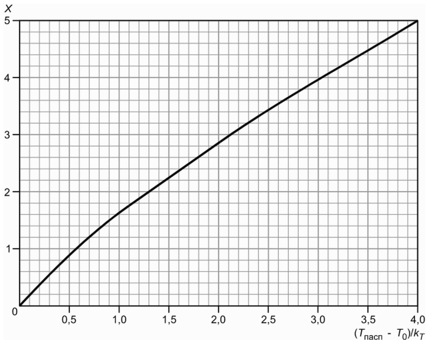
Рисунок В.2 - График для интерполяционного определения времени активации sprinklerного оросителя при термическом разрушении колбы
