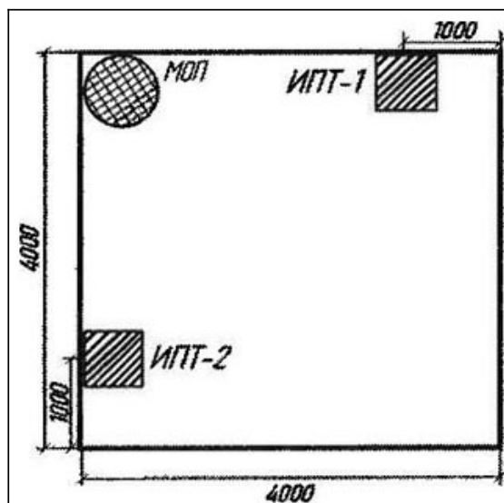
д) ИП тепловые (ИПТ-1-2)
