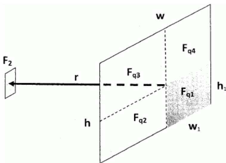
Рисунок А.3.2. Расположение излучающих поверхностей пламени
