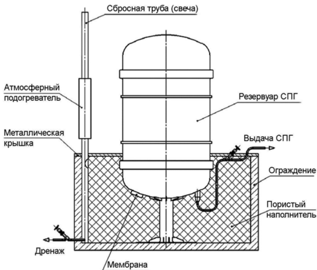
Рисунок А.1 — Принципиальная схема системы предотвращения пожара СПГ, пролитого в пределах ограждения резервуара
