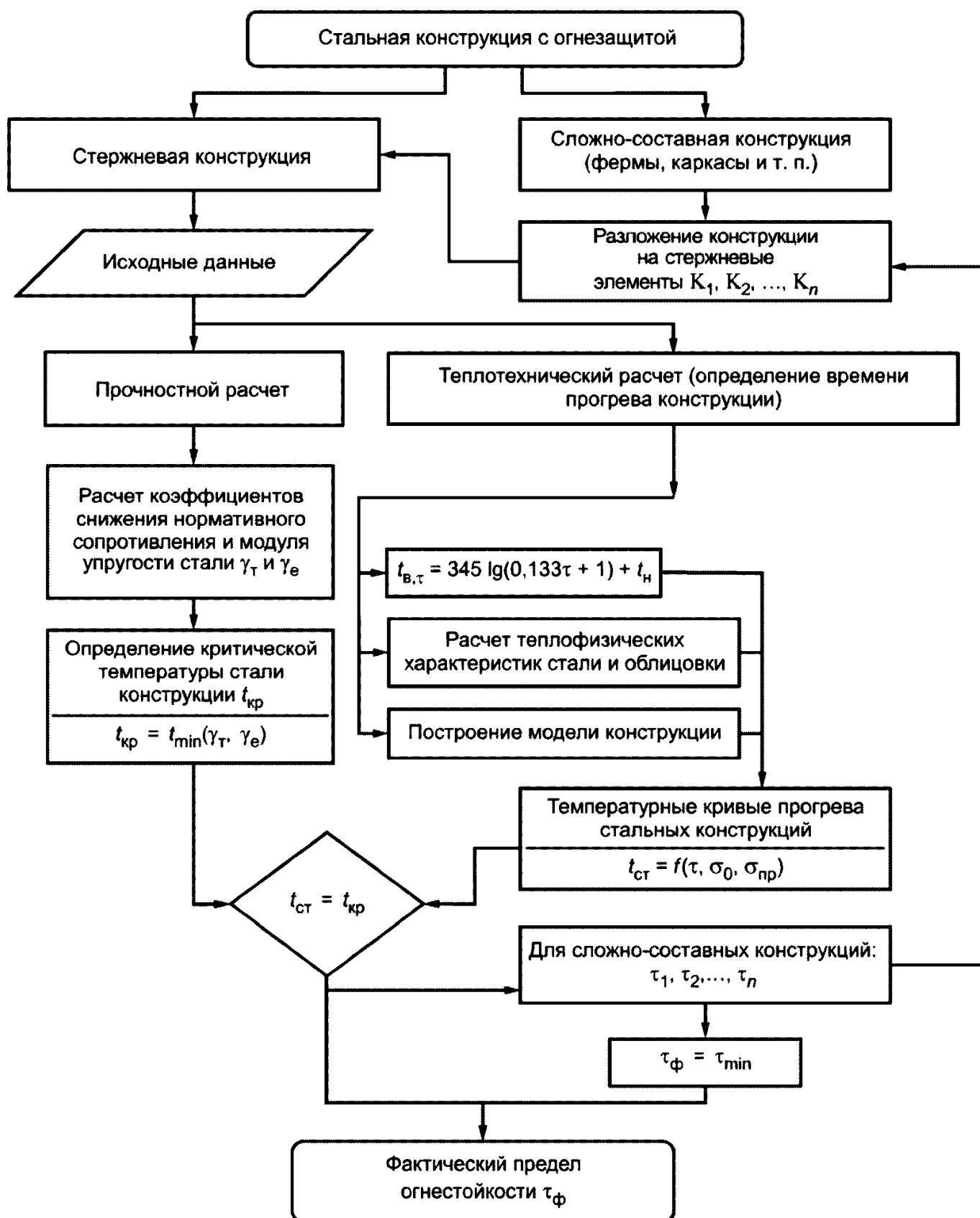
Рисунок А.1 - Алгоритм определения фактических пределов огнестойкости стальных
