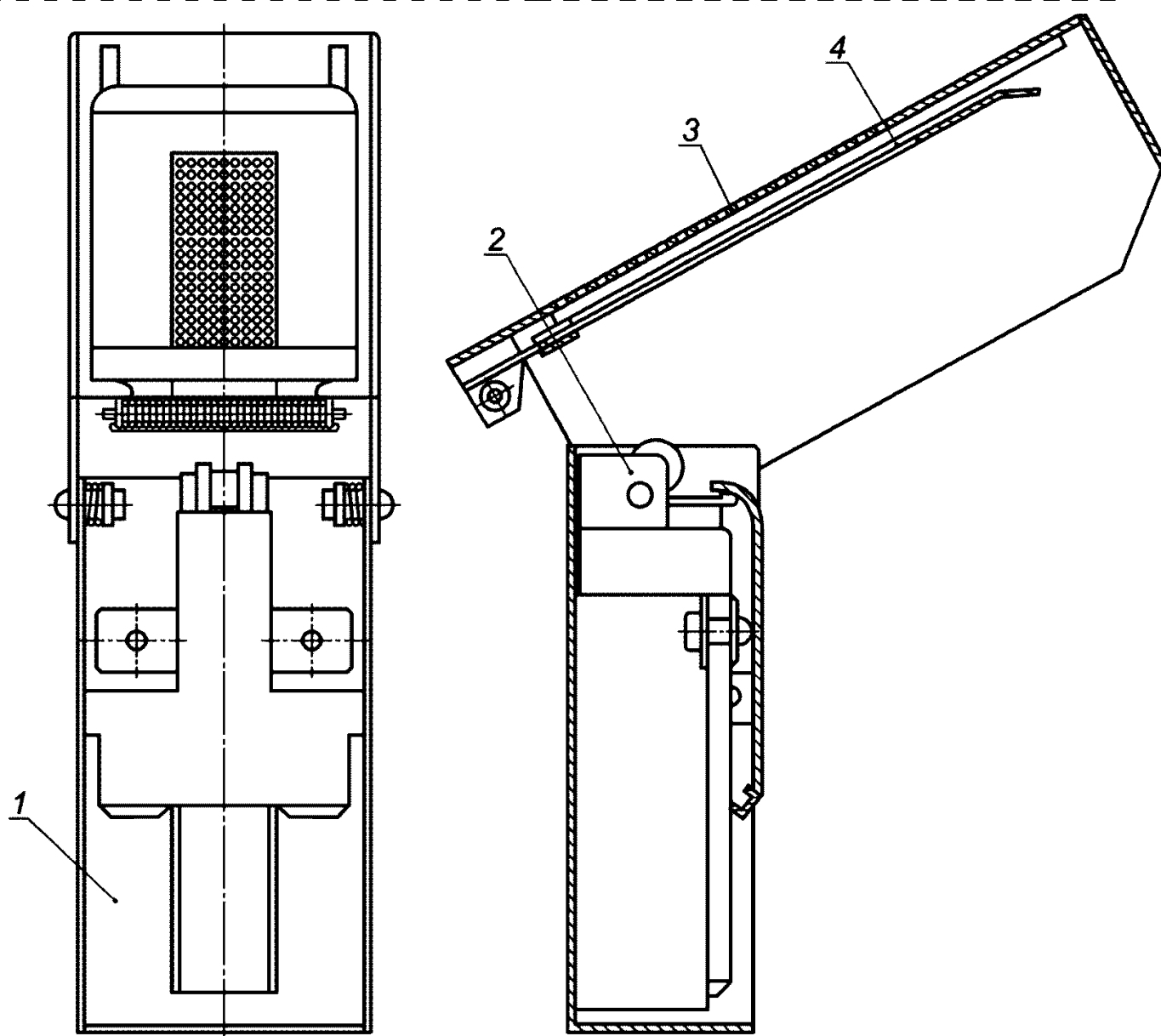
1 - корпус; 2 - газовая зажигалка; 3 - поворотная крышка; 4 - зажимное устройство
