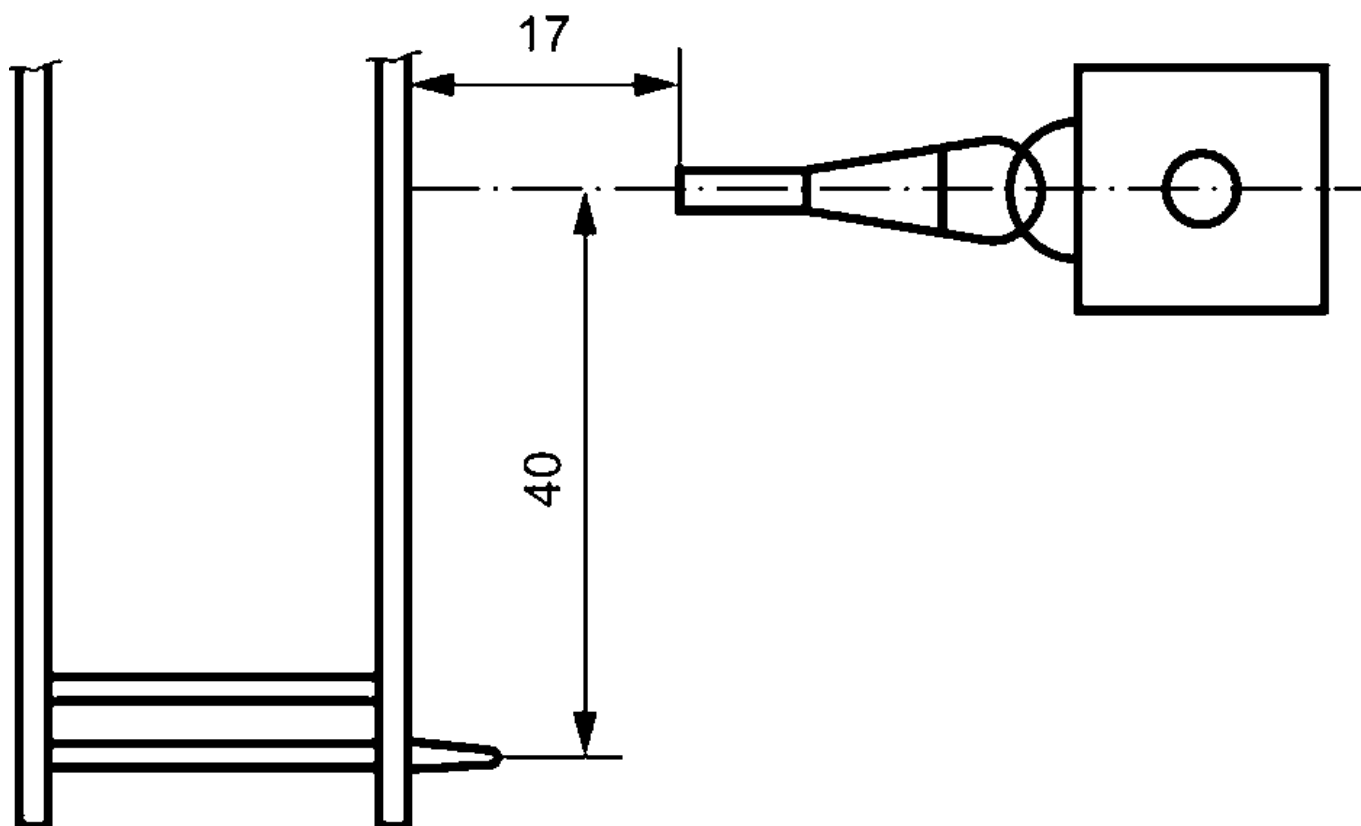
Рисунок 3 - Испытания с поверхности
