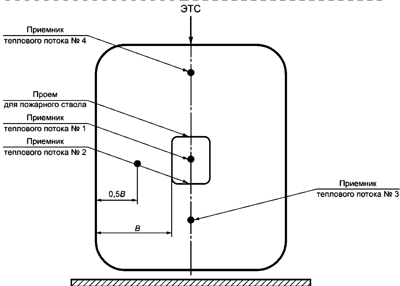
Рисунок 1 - Схема расположения приемников теплового потока
