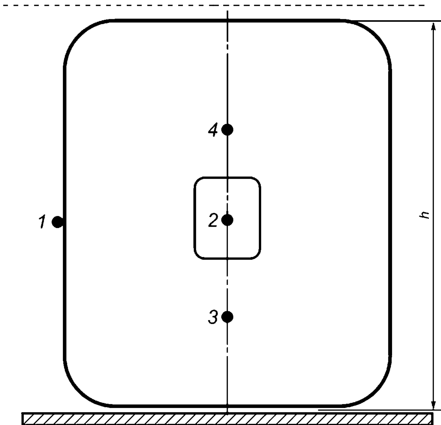
Рисунок 2 - Схема расположения приемников теплового потока на ЭТС без проема для пожарного ствола
