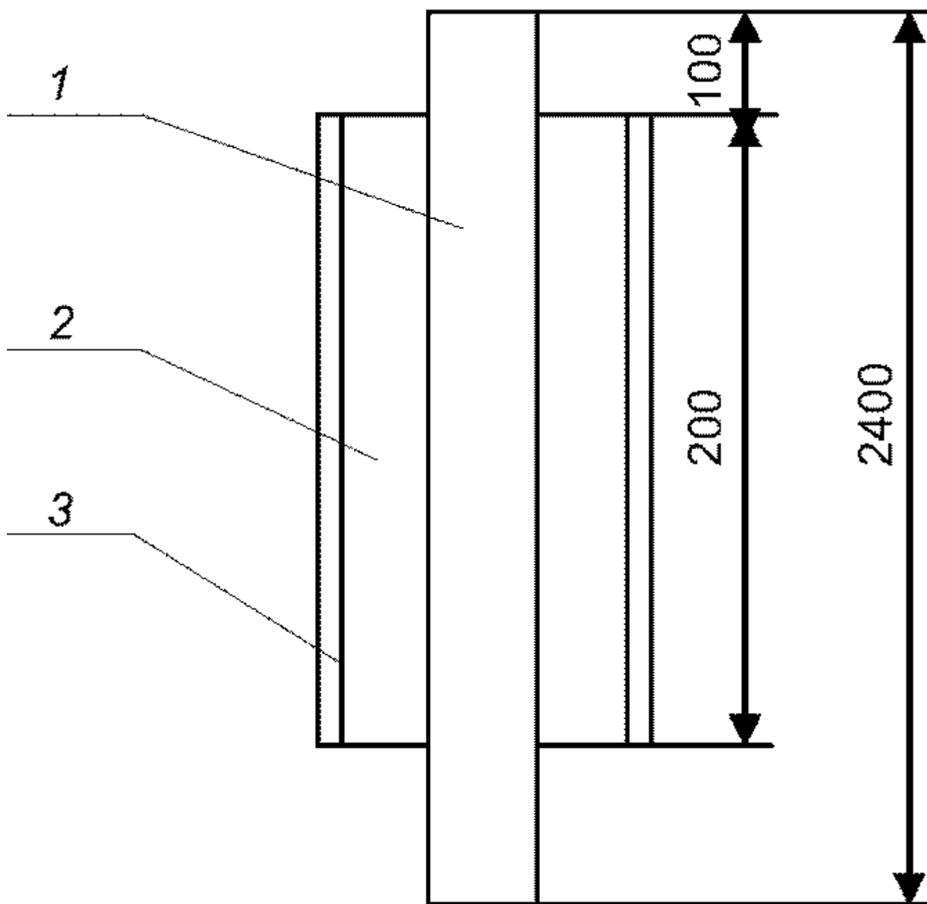
Рисунок 2. Схема калибровочной конструкции
