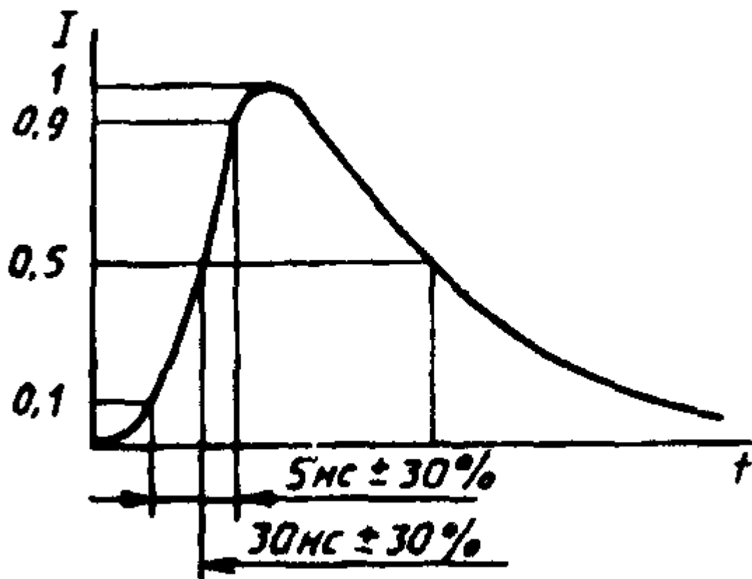
Рисунок Г.2. Форма волны
