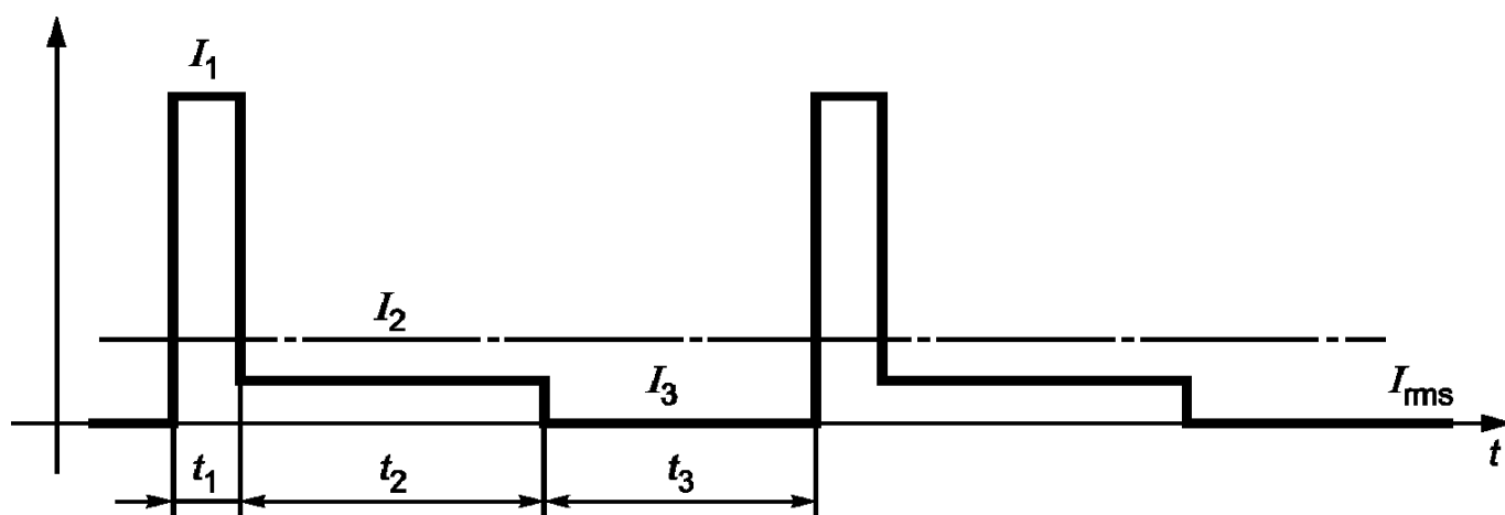
Рисунок Е.6 - Пример среднего расчета теплового эффекта
