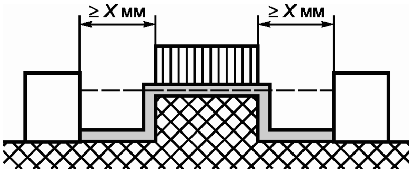
Рисунок F.1f) - Пример 5
