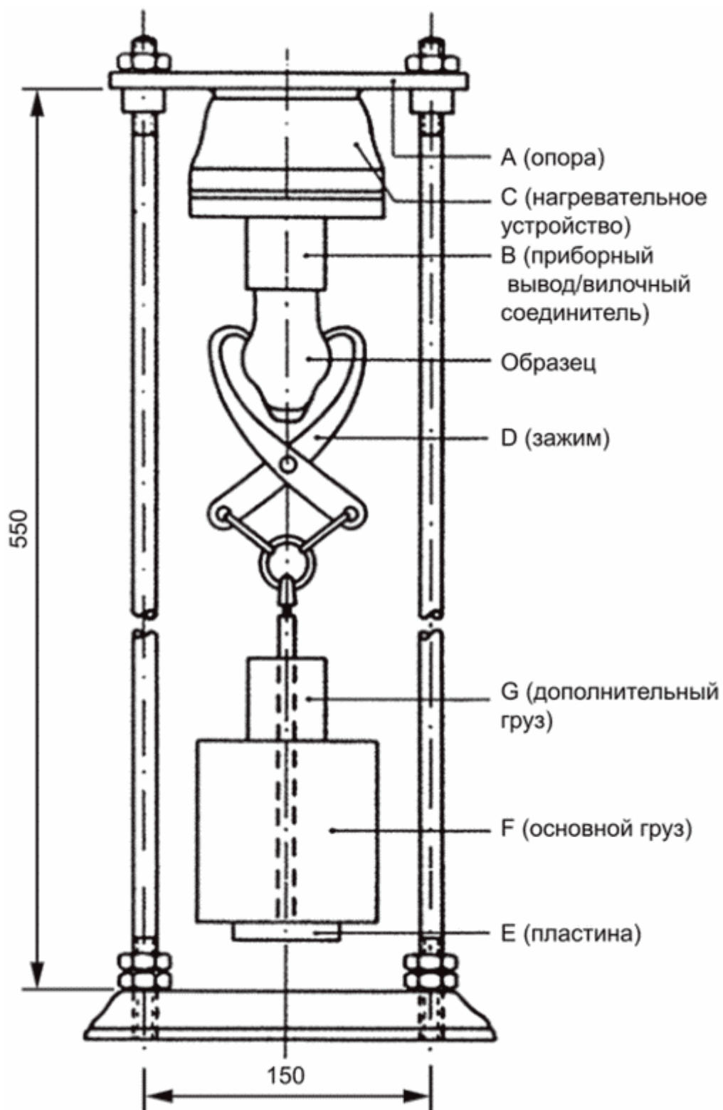
Рисунок 3 - Установка для определения максимального извлекающего усилия
