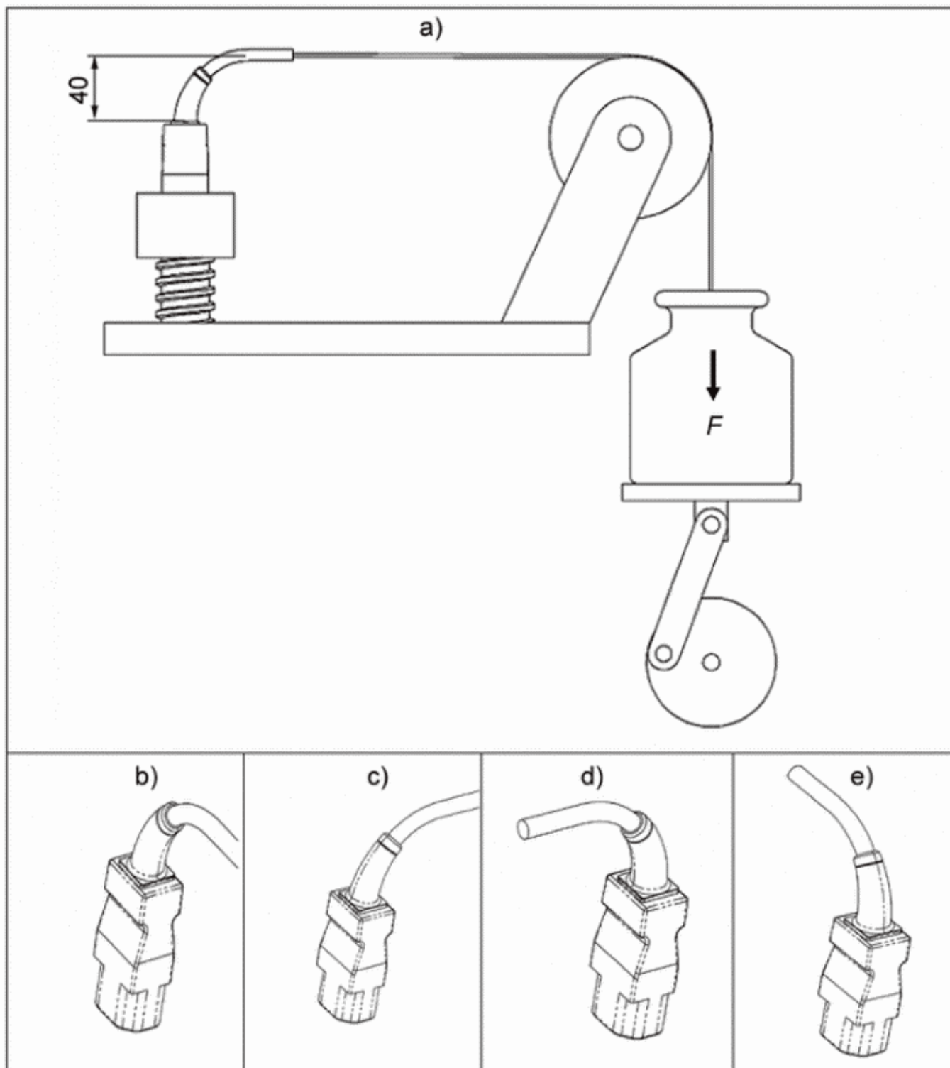
Рисунок 8 - Пример устройства для испытания на натяжение
