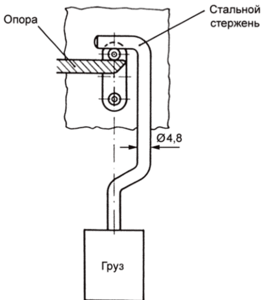
Рисунок 2 - Испытательное устройство для несплошных штырей
