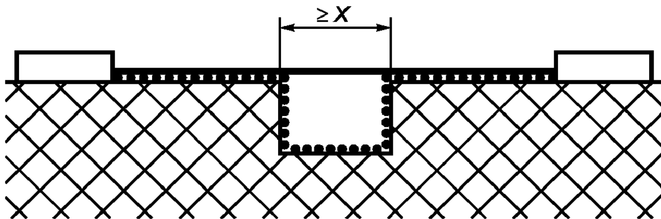
Рисунок Е.1. Узкая канавка
