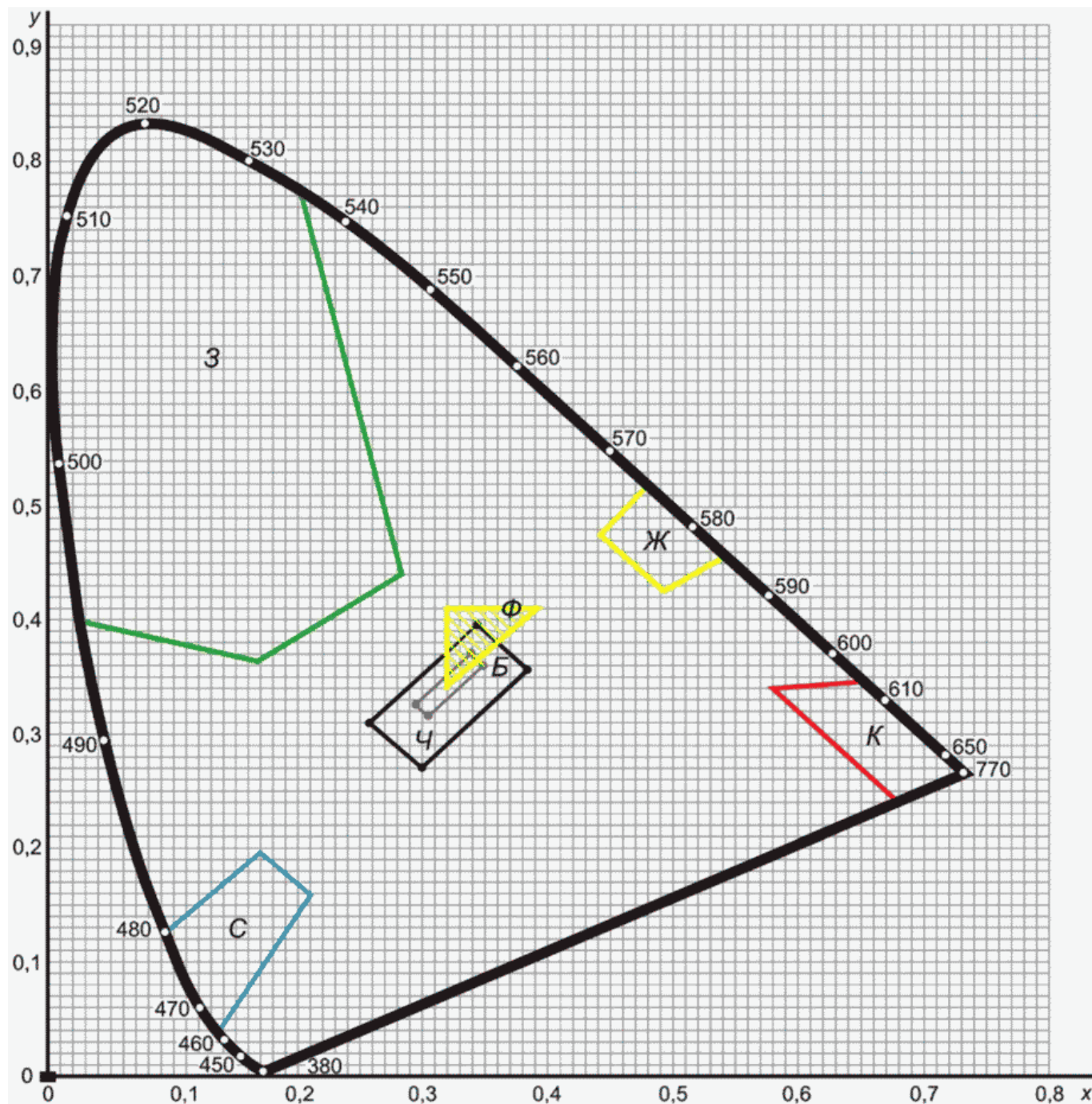
К - область красного цвета; Ж - область желтого цвета; З - область зеленого цвета; С - область синего цвета; Б - область белого цвета; Ч - область черного цвета; Ф - предпочтительная малая область для желтовато-белого фосфоресцирующего цвета Рисунок Б.1 - Допустимые области цветности сигнальных и контрастных цветов элементов ФЭС, знаков безопасности и сигнальной разметки на локусе цветности x, y МКО 1931 г.
