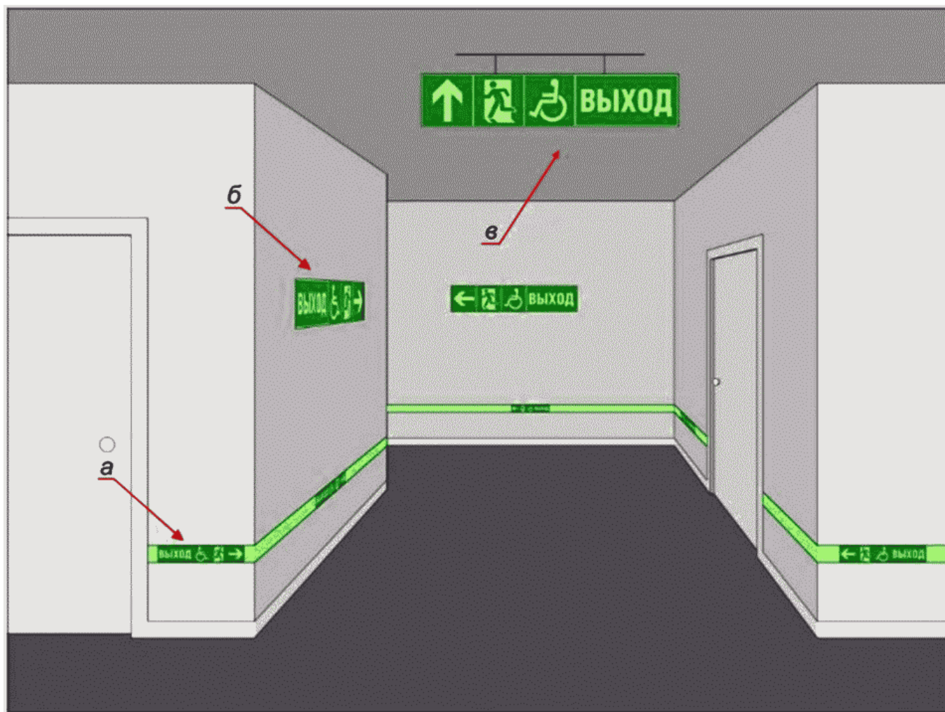
а - низко расположенная настенная направляющая линия с включенным в ее состав указателем направления эвакуации; б - настенный комбинированный указатель направления эвакуации; в - подвесной комбинированный указатель направления эвакуации Рисунок В.8 - Пример обозначения совмещенного основного пути эвакуации и пути эвакуации для инвалидов-колясочников в коридорах, проходных помещениях и т.п.
