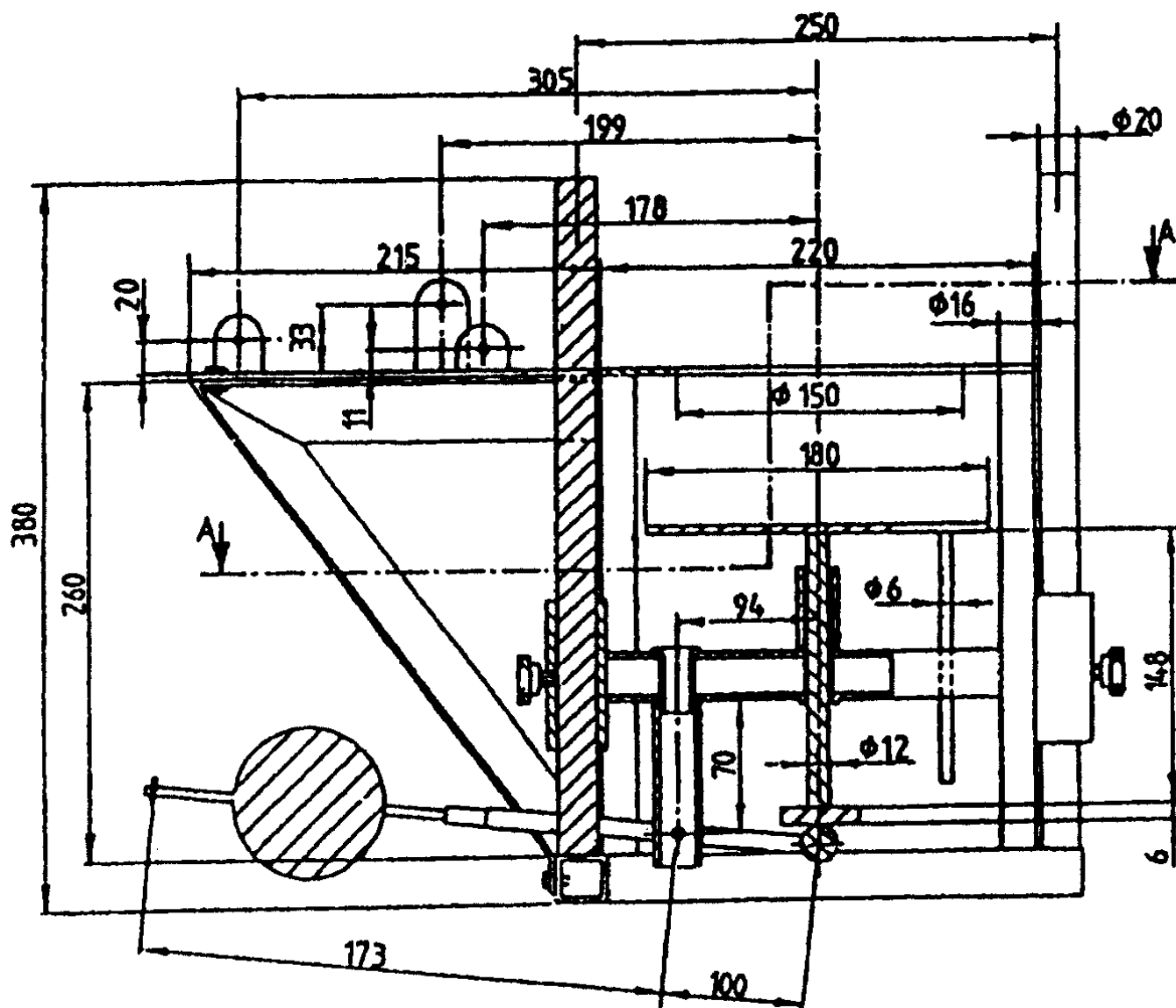
Рисунок А2. Опорная станина (разрез по ВВ)
