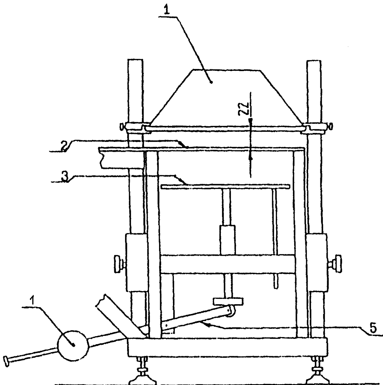
Рисунок А3. Опорная станина (разрез по АА)
