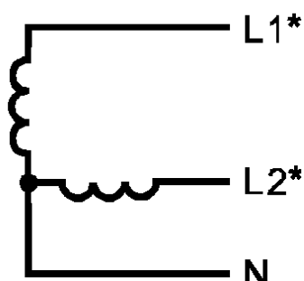
Рисунок 2. Однофазная трехпроводная электрическая цепь
