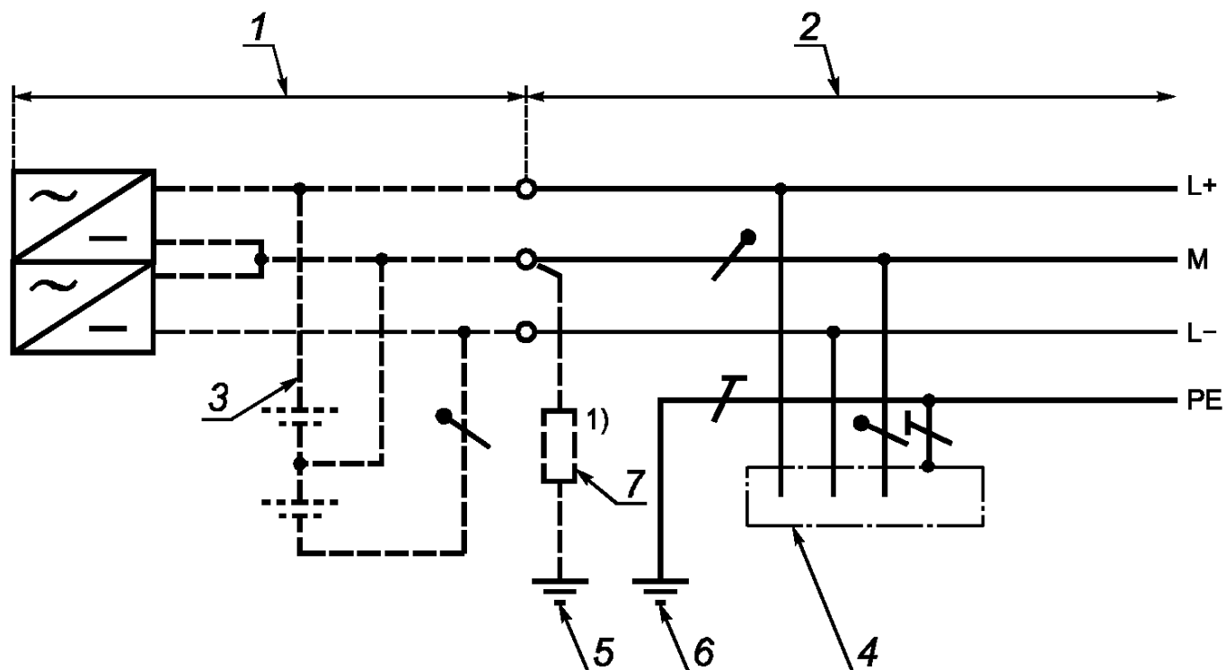
Тип b) - трехпроводная система
