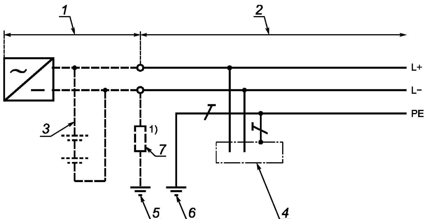
Тип b) - трехпроводная система
