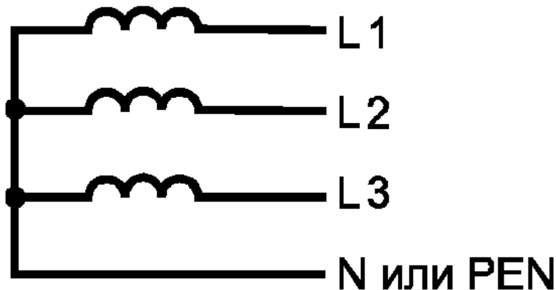
Рисунок 5. Трехфазная четырехпроводная электрическая цепь
