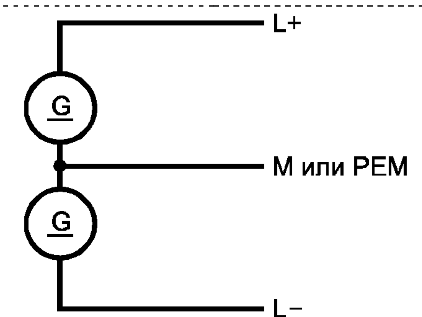
Рисунок 7. Трехпроводная электрическая цепь
